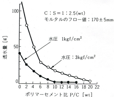
第1図 スチレン・ブタジエン合成ゴムラテックスを混入したポリマーセメントモルタルの透水性
