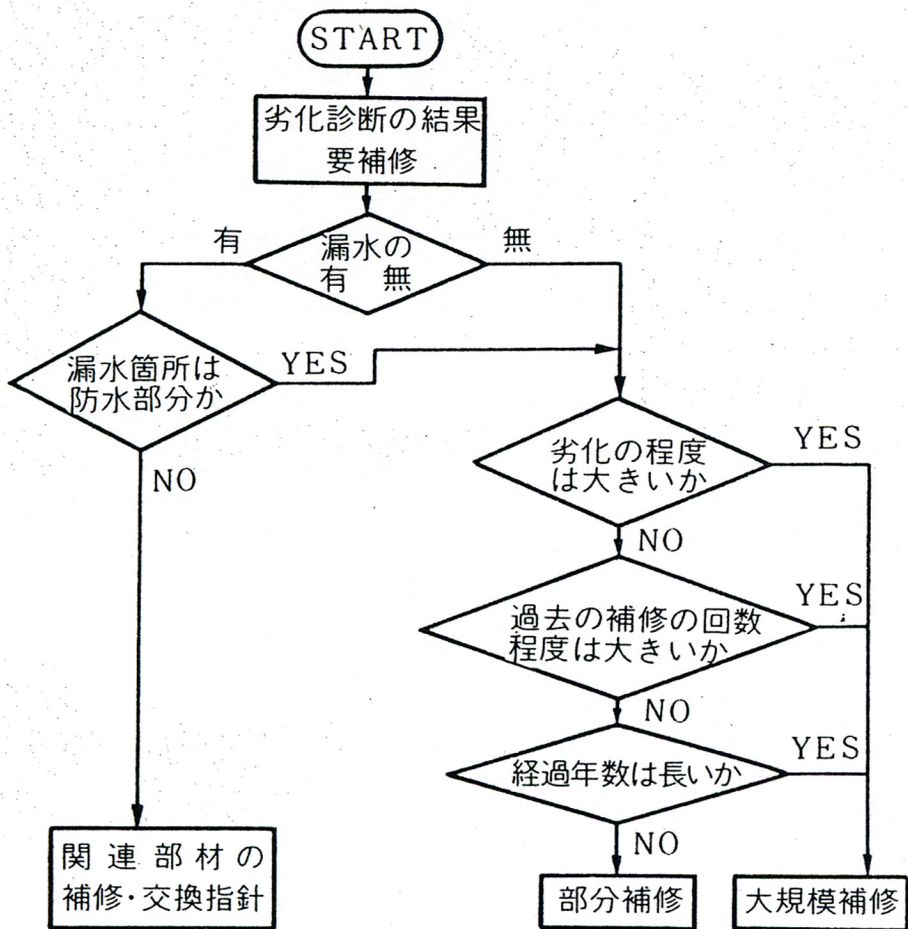
第1図 屋根メンブレン防水の補修規模判定フロー
