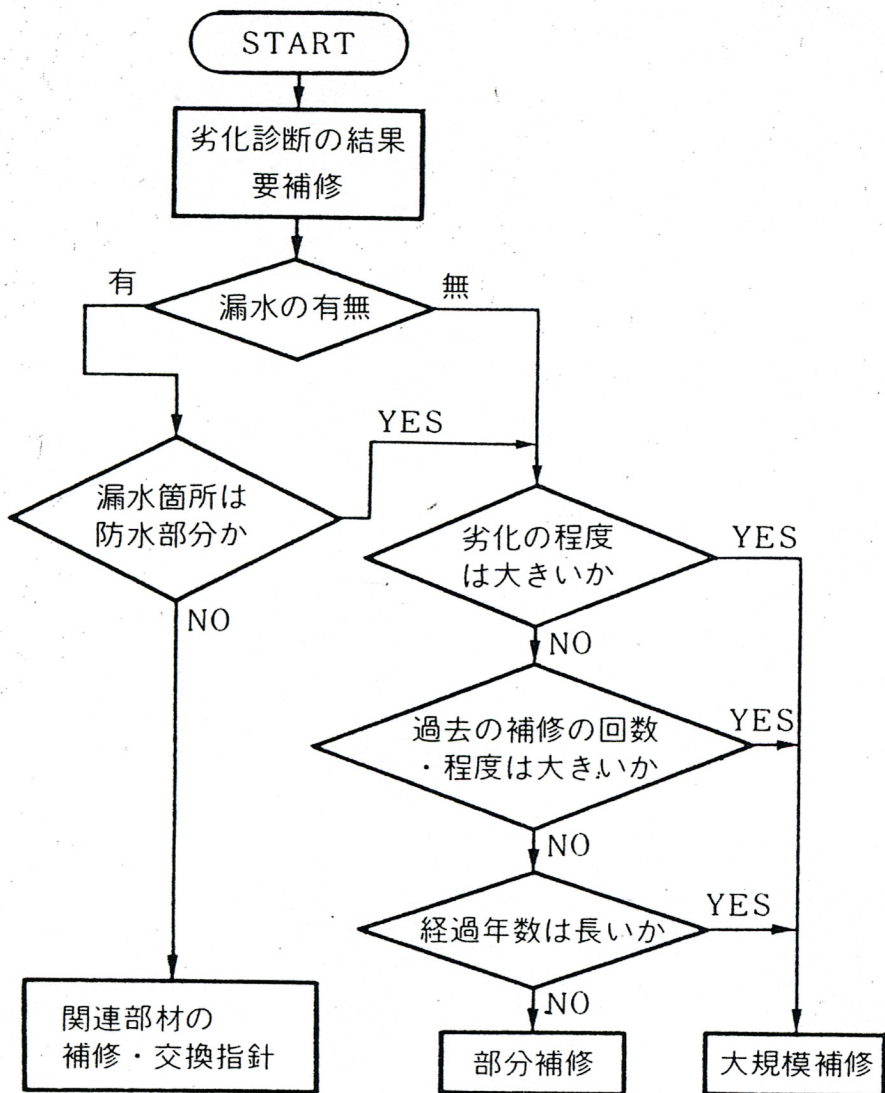
第 1 図 屋根メンブレン防水の補修規模判定フロー
