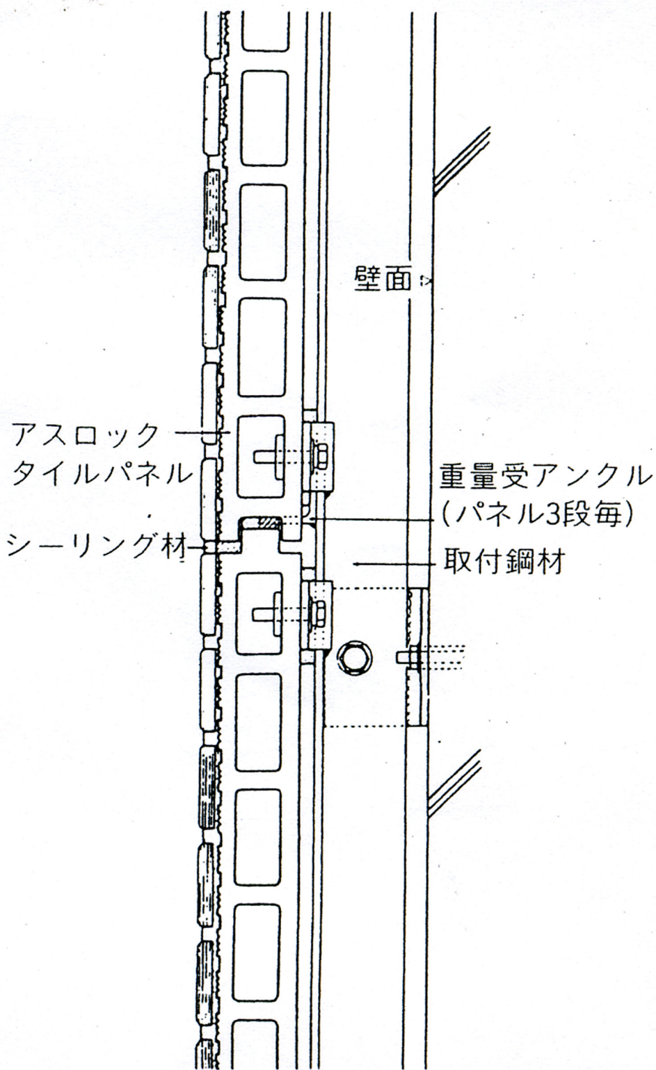
断面詳細例
