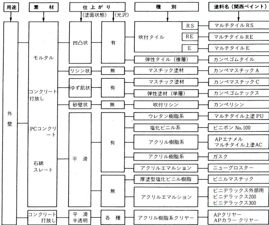
第2図 建築塗装システム〔外部〕(関西ペイントの例)
