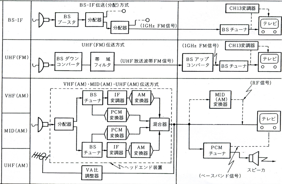
第1図 衛星放送受信システム
