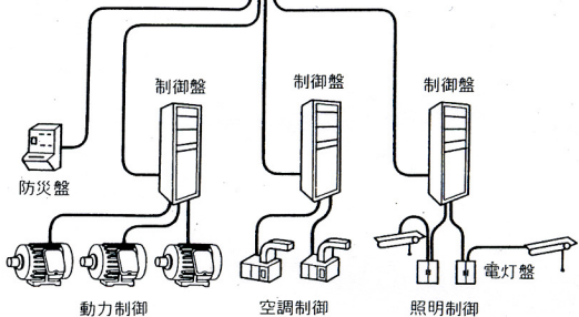
第2図 分散制御システム
