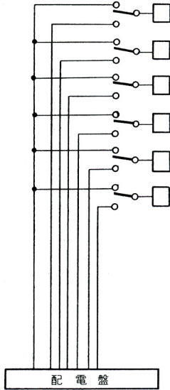
第3図 二重幹線系統の例
