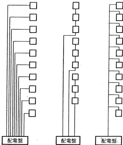
第2図 一般的幹線系統例
