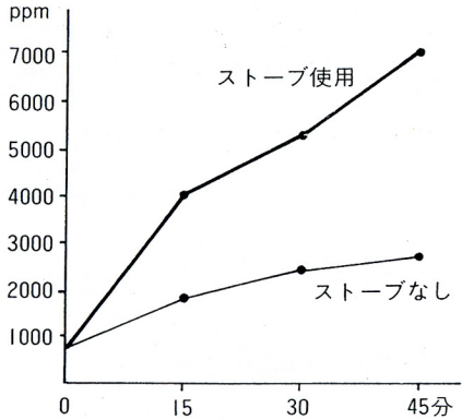
開放型石油ストーブ使用時のCO 2 発生量
