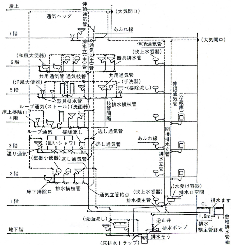
排水通気管系統図
